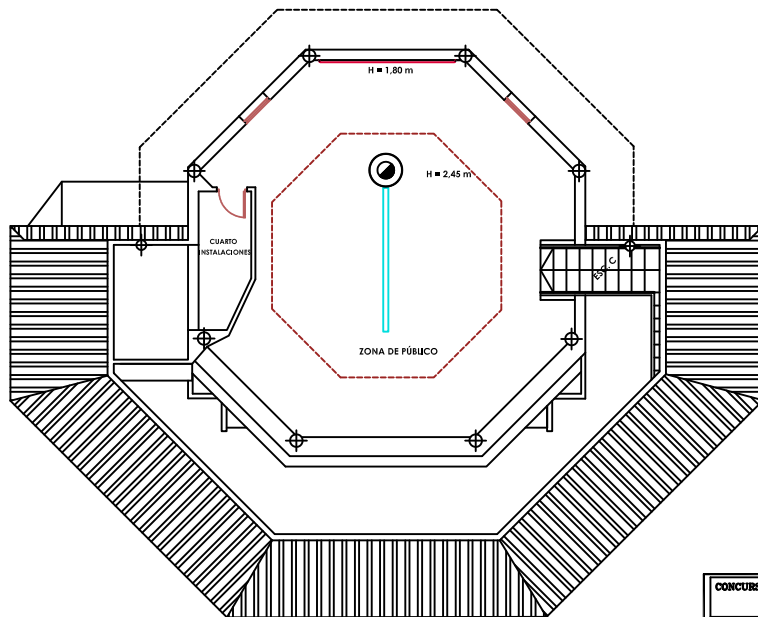
PLANTA ALTA
